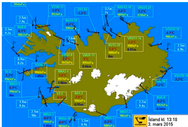
Mynd 9. Dæmi um rauntímaupplýsingar úr upplýsingakerfi Vegagerðarinnar. Hvitir kassar með hvítum tölum sýna hæð kenniöldu í metrum og meðalsveiflutíma í sekúndum.
