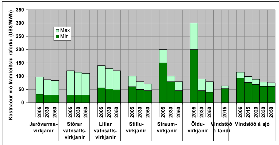
Mynd 16. Áætluð þróun í framleiðslukostnaði grænnar orku byggð á jafnaðartölum IEA.
