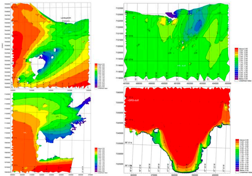
Mynd 12. Ölduspár af hafi færðar inn á firði, flóa og strandsvæði, efst til vinstri og réttisælis, strandsvæðið milli Vestmannaeyja og lands, strandsvæðið utan við Hornafjarðarós, Skjálfandinn og Faxaflói.
