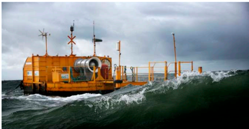
Fljótandi vatnsúlu sveiflu virkjun frá Ocean Energy Limited http://www.oceanenergy.ie
