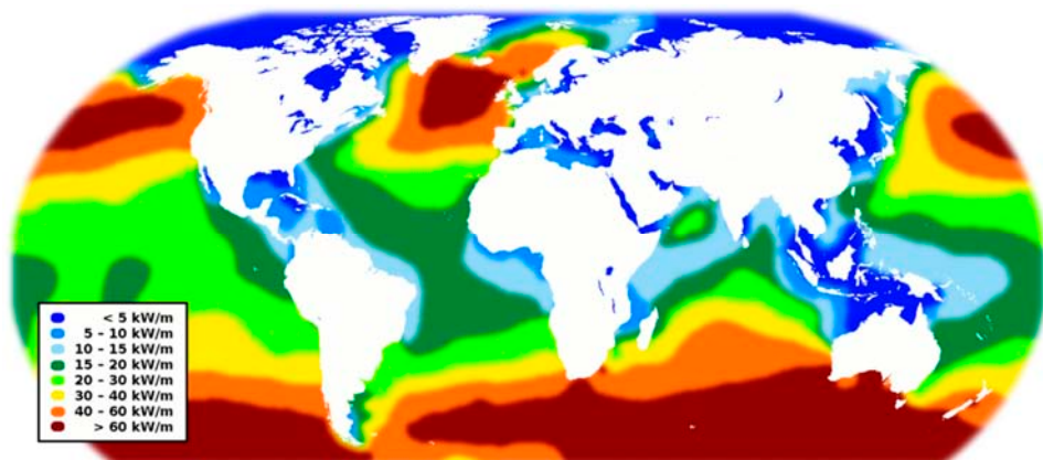
Mynd 8 Heimskort sem sýnir meðalafl í öldum sem kW á lengdarmetra öldu. ( http://commons.wikimedia.org/wiki/File:World_wave_energy_resource_map.png )
