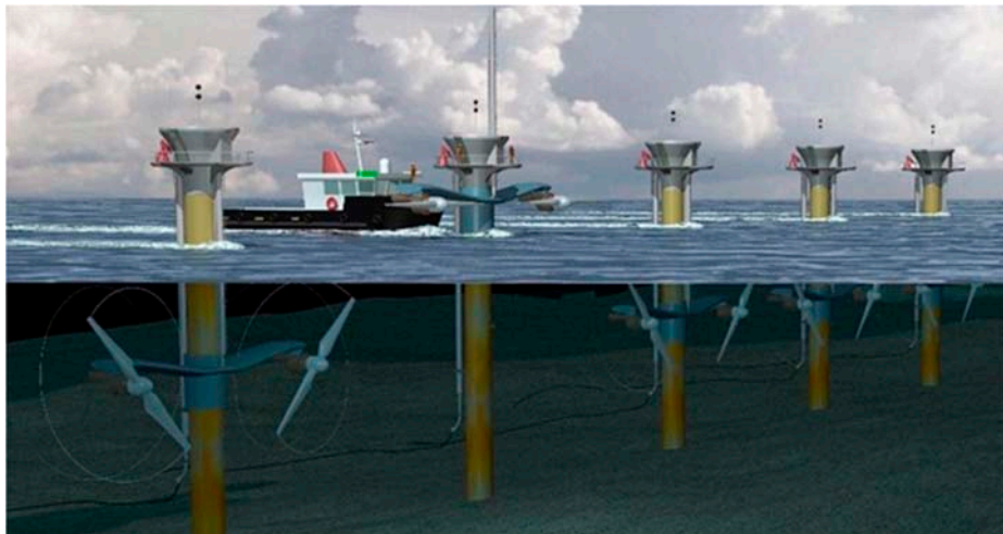
Simens MCT ( http://www.marineturbines.com/ )
