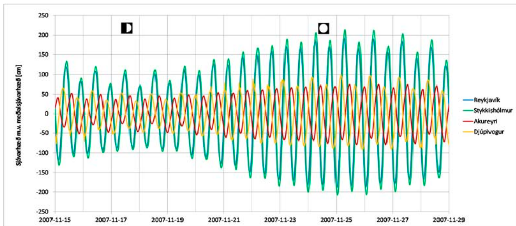
Mynd 1. Reiknuð sjávarhæð í Reykjavík, Stykkishólmi, Akureyri og Djúpvogum.
