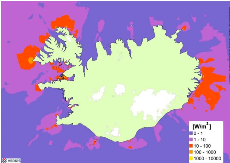
Mynd 6. Reiknað hámarksafli sjávarfalla á stórstreymi (W/m 2 ).
