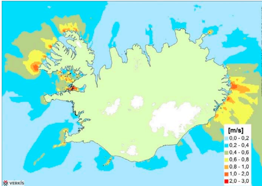
Mynd 4. Reiknaður hámarks straumhraði sjávarfalla á stórstreymi.
