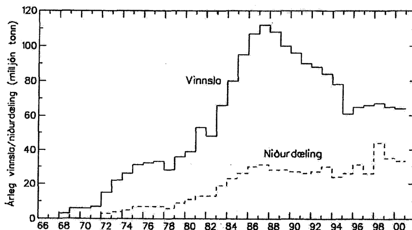
Mynd 3. Vinnslusaga Geysers-jarðhitakerfisins í Kaliforníu
