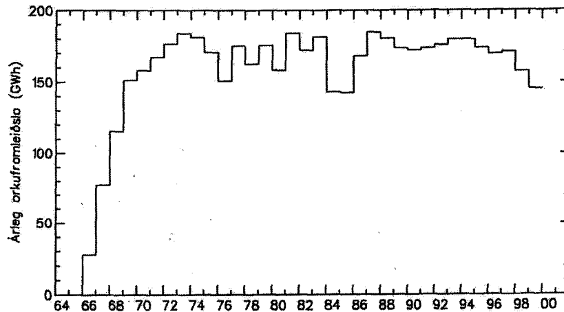
Mynd 1. Vinnslusaga jarðhitakerfisins í Matsukawa í Japan.
