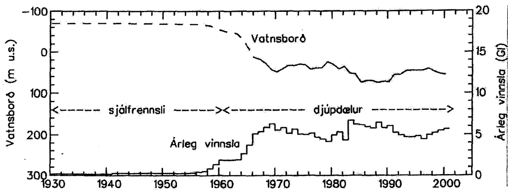
Mynd 2. Vinnslusaga jarðhitakerfisins í Laugarnesi í Reykjavík.
