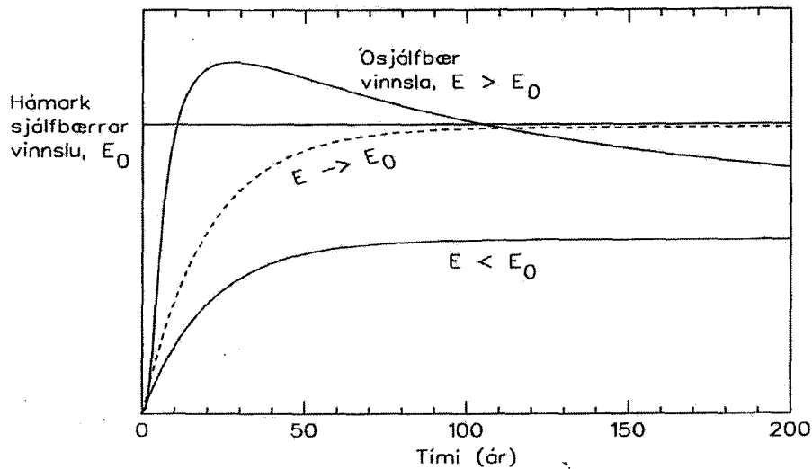
Mynd 4. Skýringarmynd fyrir hugtakið sjálfbær vinnsla jarðhita.
