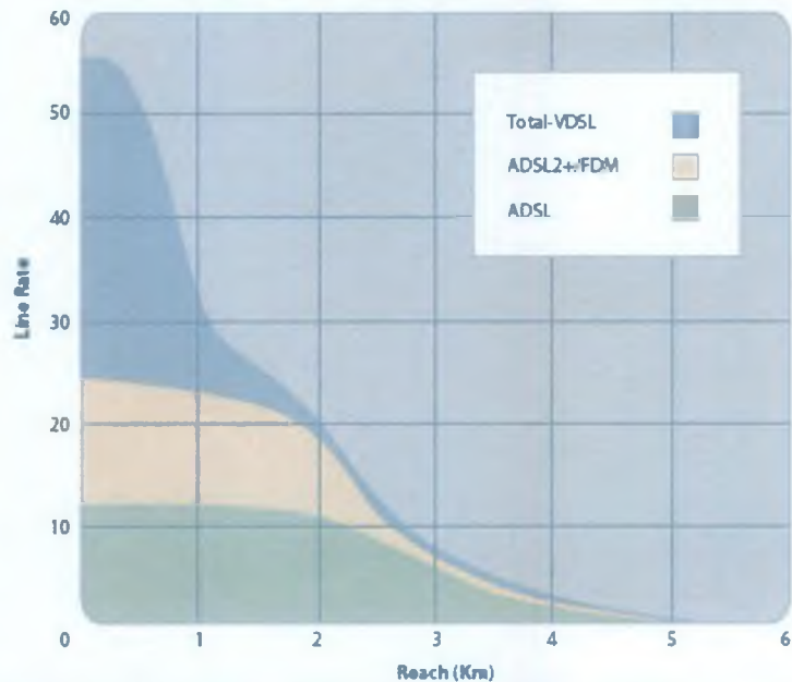
Mynd 1. Samhengi fjarlægðar frá sírstöð til notanda og gagnaflyttingshraða (mb/s) mismunandi tenginga
