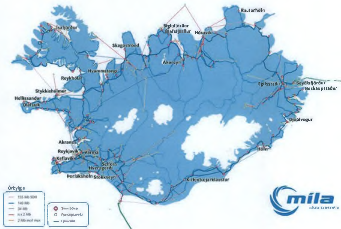
Mynd 2. Ljósleiðarakerfi Milu
